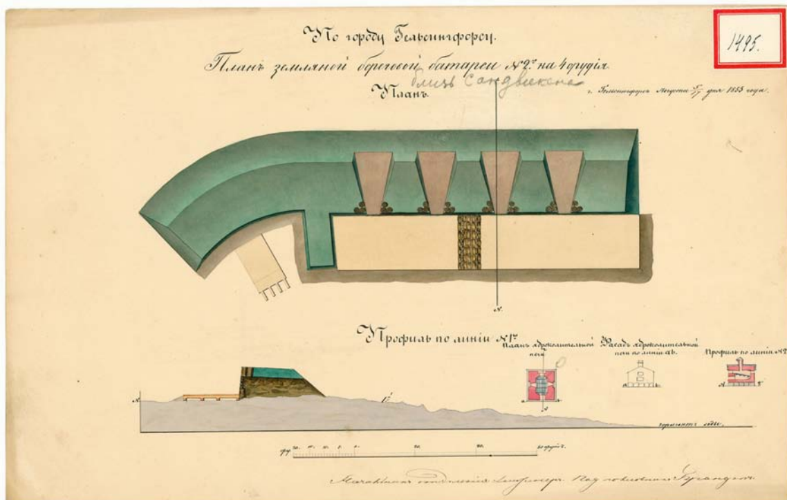
Suunnitelma Hietalahden patterista vuodelta 1855
